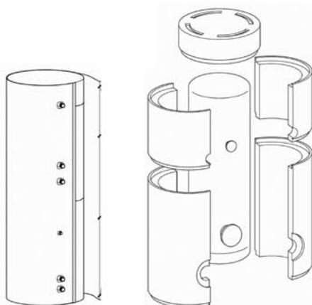
Монтаж обшивки
